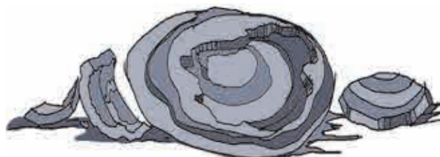
Fig. 2.8 : Exfoliation
