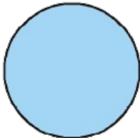
A circle
