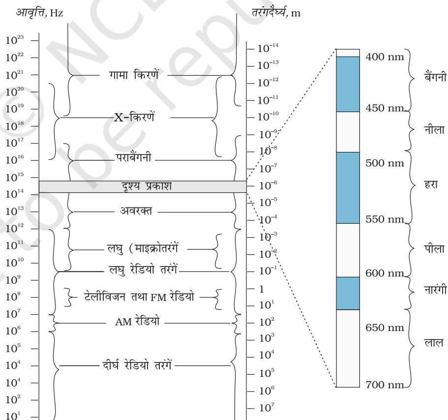
चित्र 8.5 वैद्युतचुंबकीय स्पेक्ट्रम जिसके विभिन्न भागों के सामान्य नाम दर्शाए गए हैं। विभिन्न भागों के बीच कोई स्पष्ट विभाजन रेखा नहीं है।
