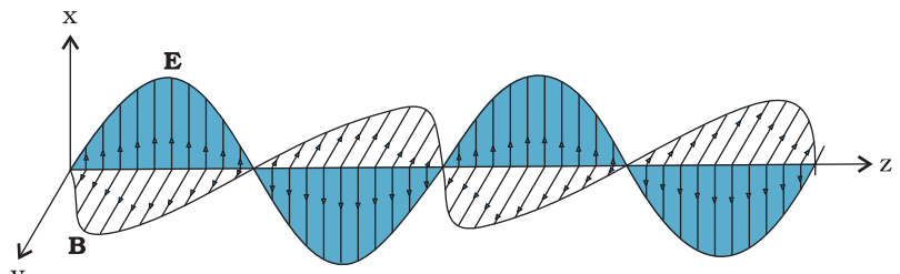
चित्र 8.4 एक रेखीय ध्रुवित वैद्युतचुंबकीय तरंग जो z -दिशा में गमन कर रही है और जिसका दोलनकारी विद्युत क्षेत्र \mathbf{E} , x -दिशा के अनुदिश एवं दोलनकारी चुंबकीय क्षेत्र \mathbf{B} , y -दिशा के अनुदिश है।
