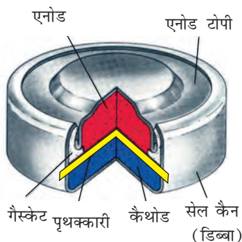
चित्र 3.9—सामान्यतः प्रयुक्त मर्क्युरी सेल, जिनके अपचायक तथा मर्क्युरी (II) ऑक्साइड ऑक्सीकारक हैं।
