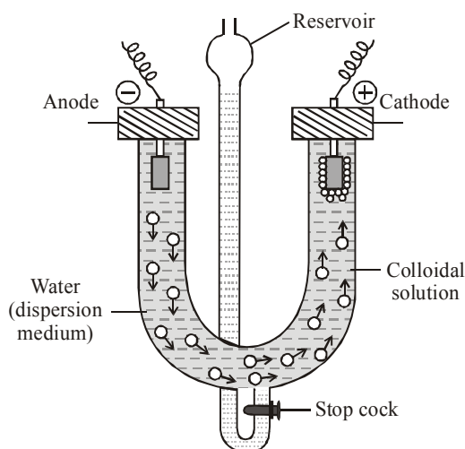
Fig. : Electrophoresis
